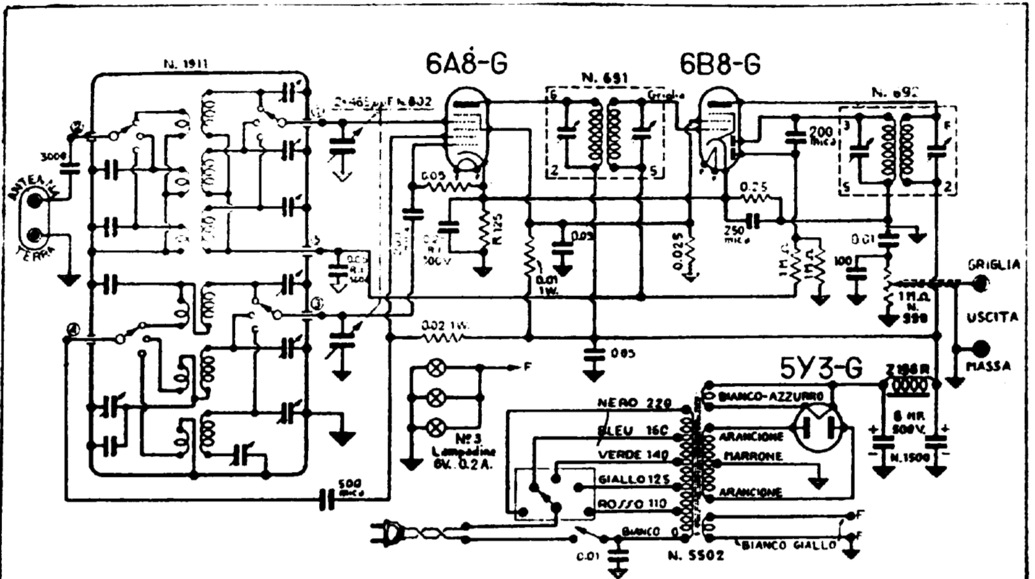
SINTONIZZATORE SUPER G.38 PER AMPLIFICATORI ONDE CORTE-MEDIE-LUNGHE
